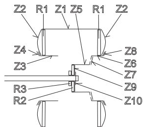
ZADNÉ KOLESO
