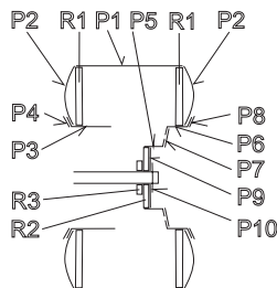
PREDNÉ KOLESO
